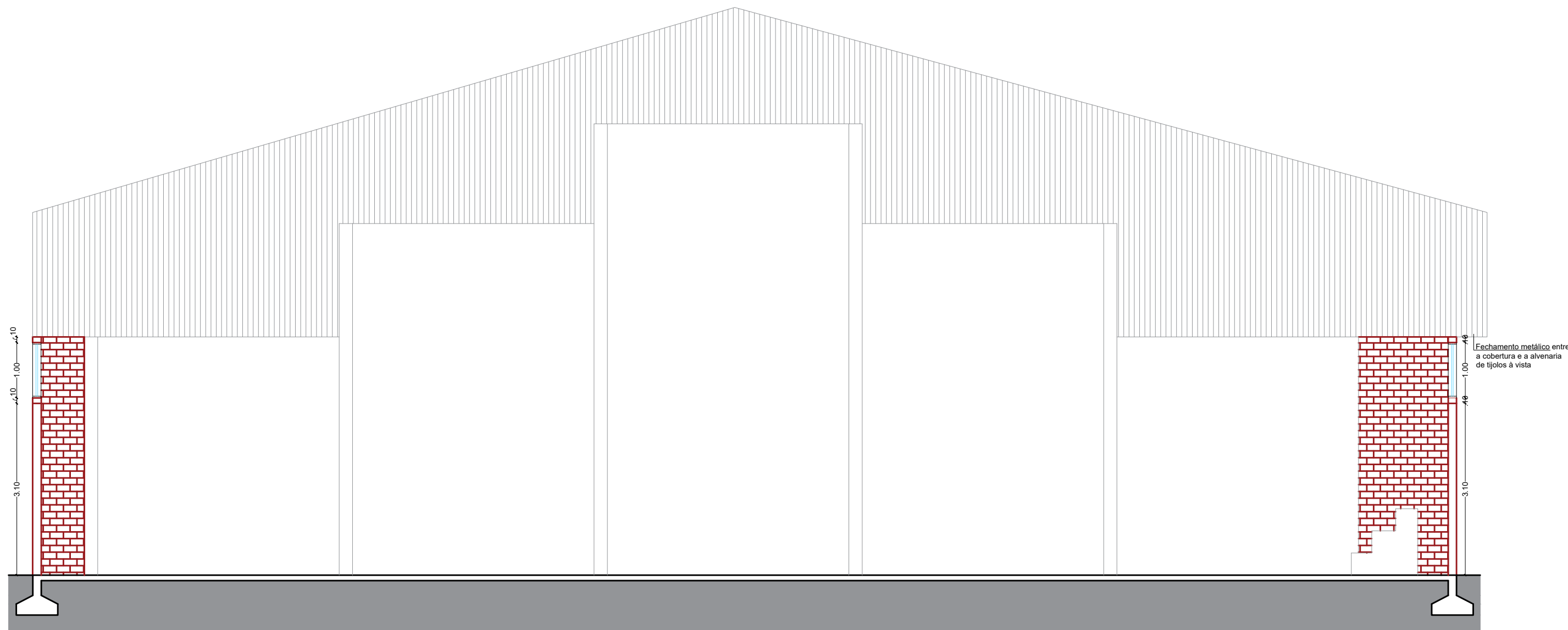
Corte AA Esc.: 1/75
